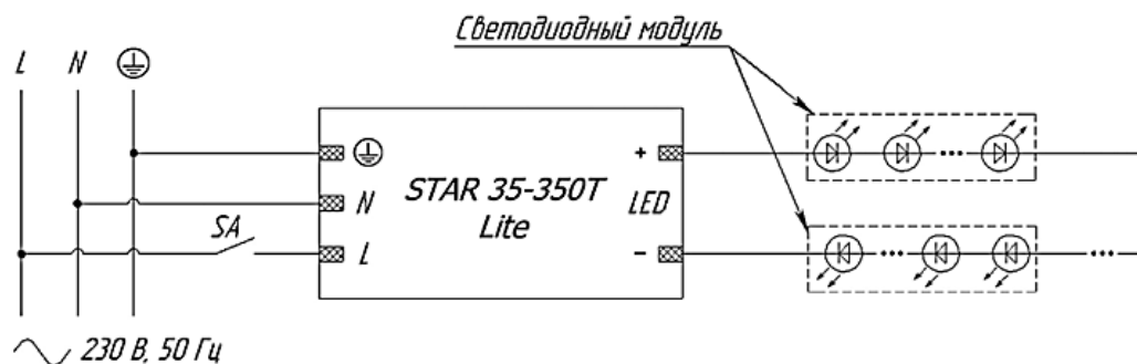
б) Схема последовательного соединения светодиодных модулей
