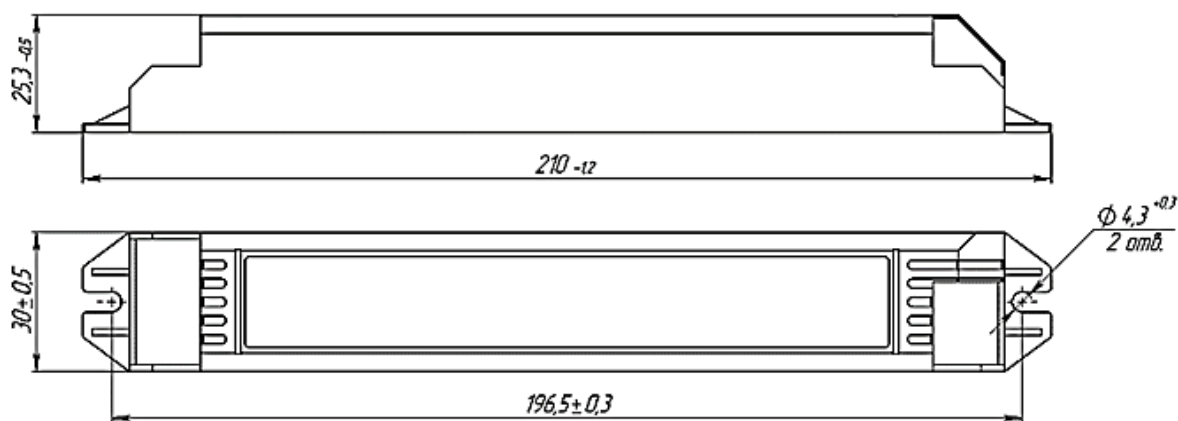
Рисунок 1 – Габаритные и установочные размеры
